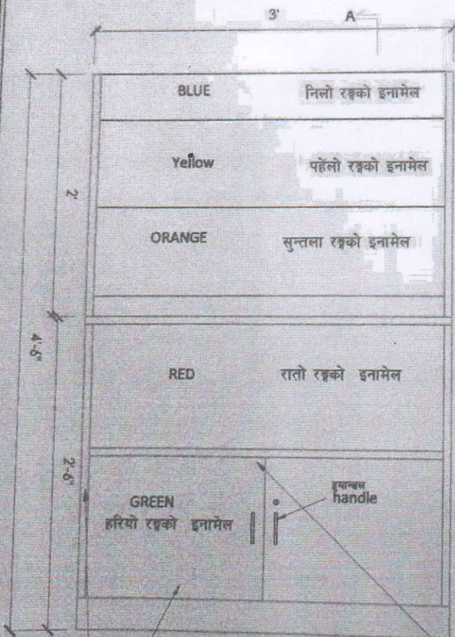
साथिको मोहोडा (Plan)
